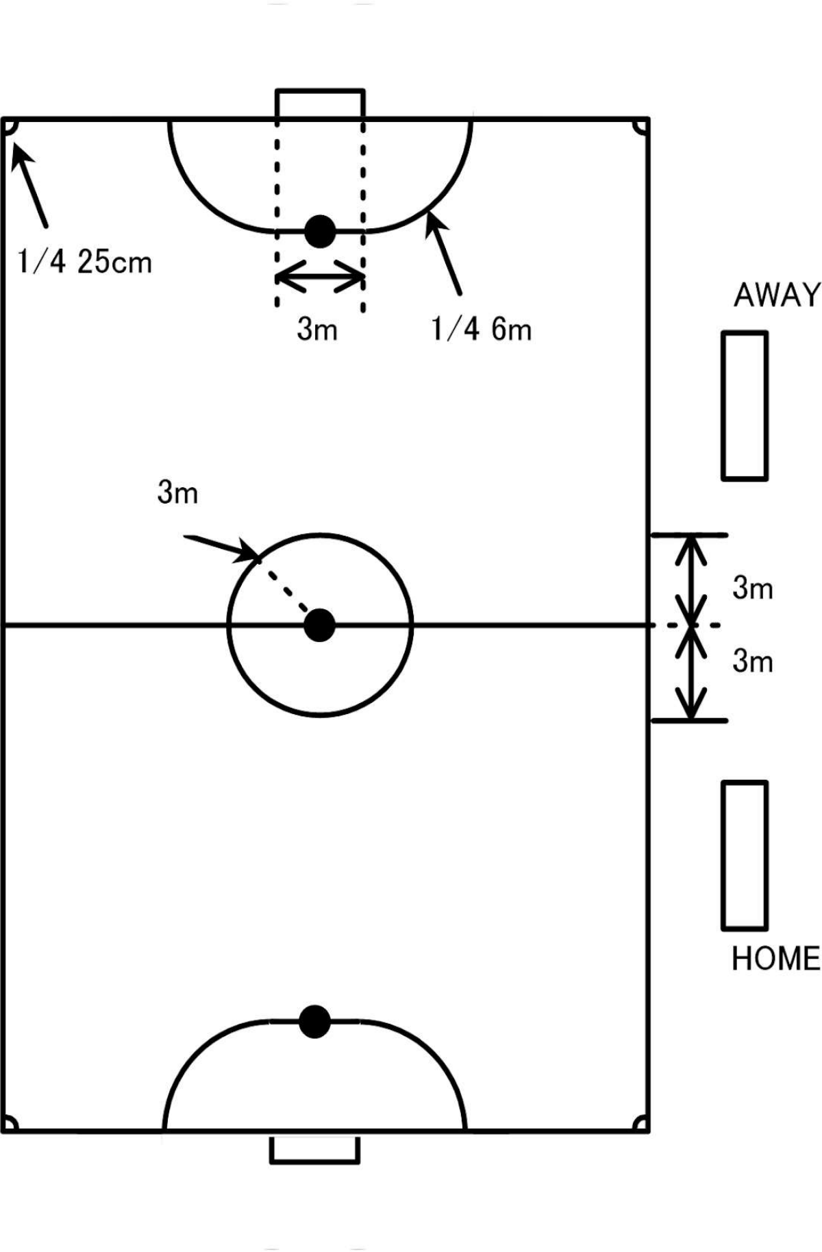
コート寸法参照図
